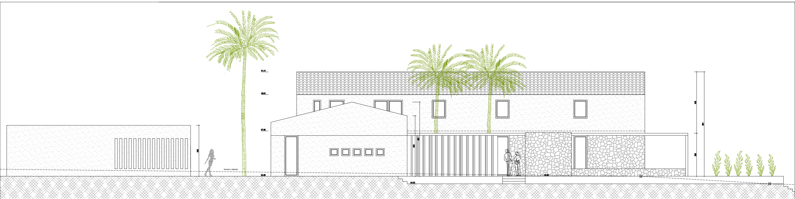
ALZADO SUROESTE
