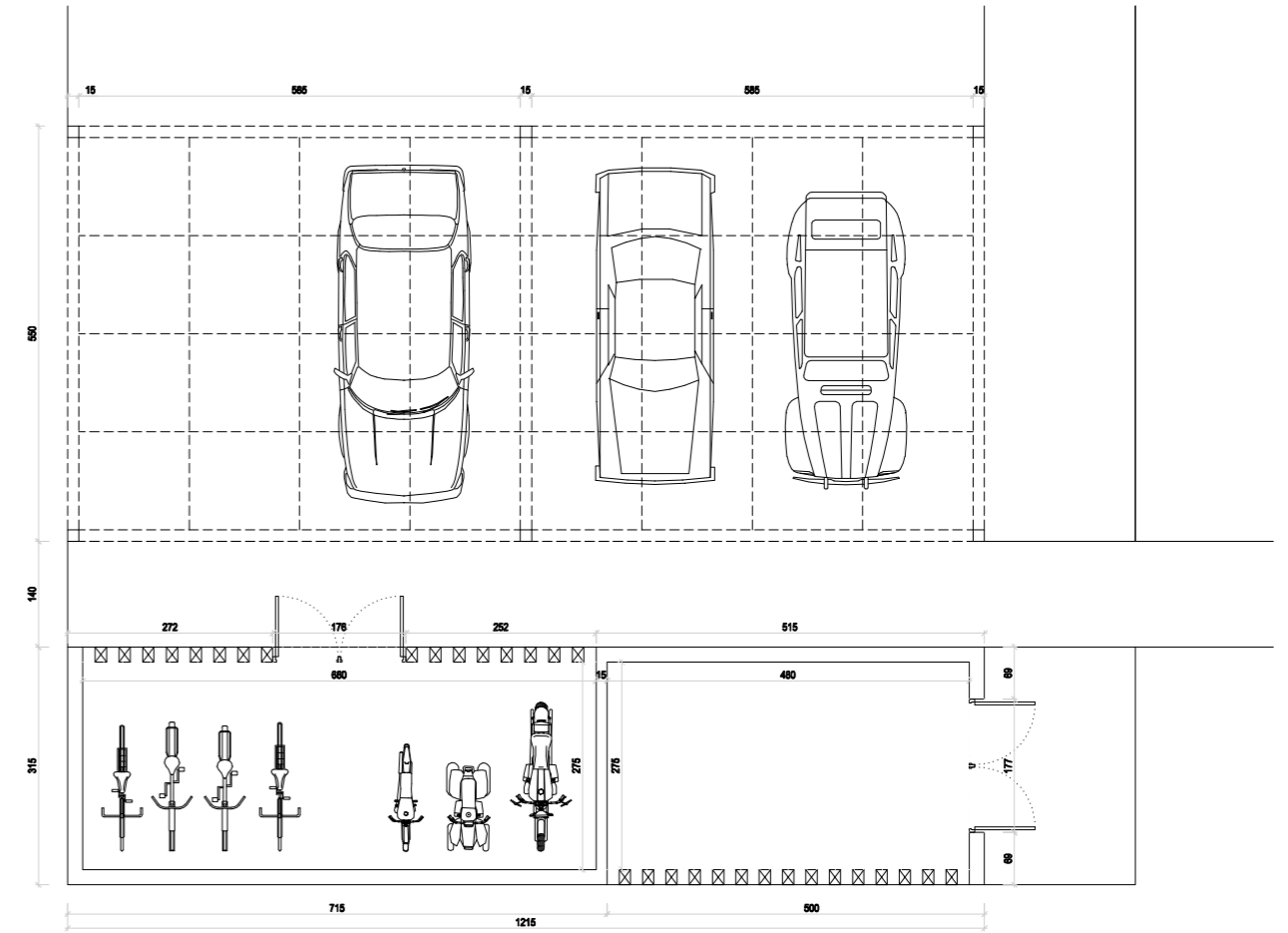
COTAS
