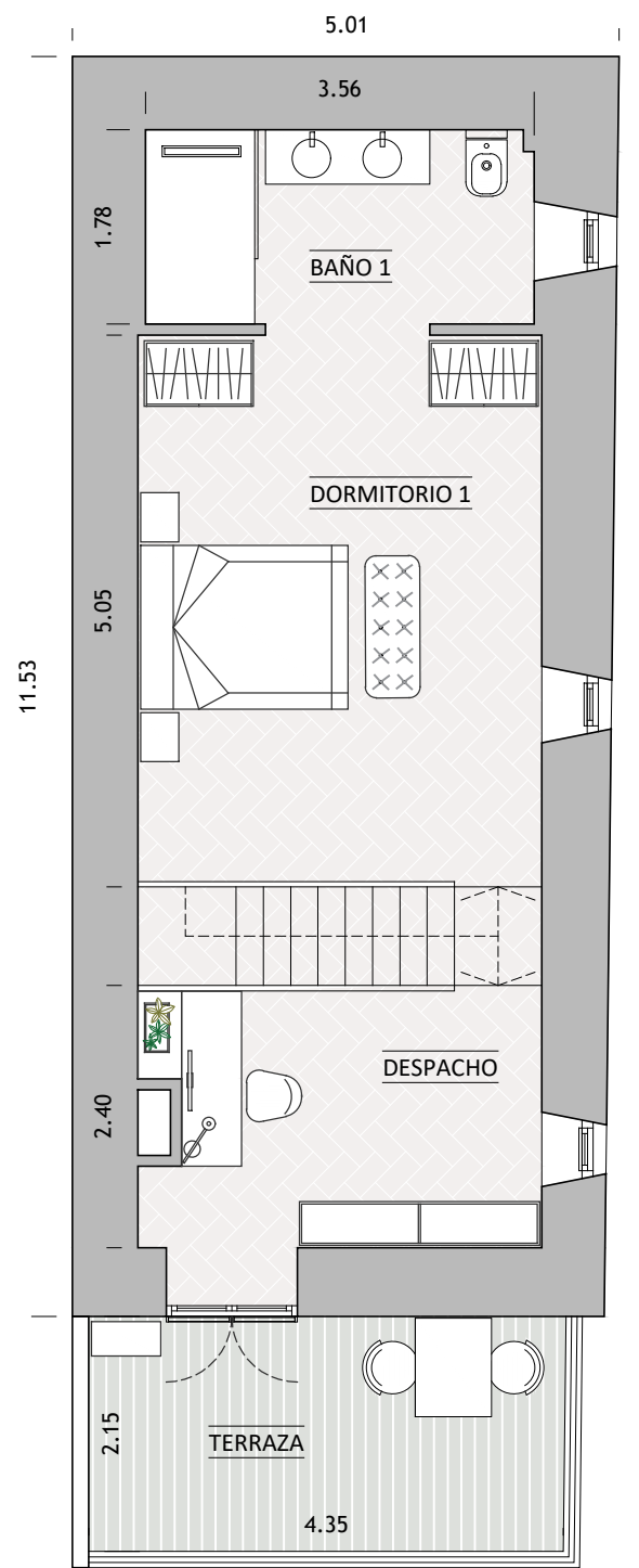
PLANTA PRIMERA
