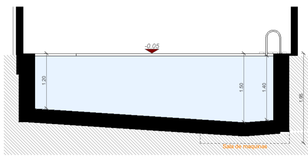
Sección D-D' 1:50
