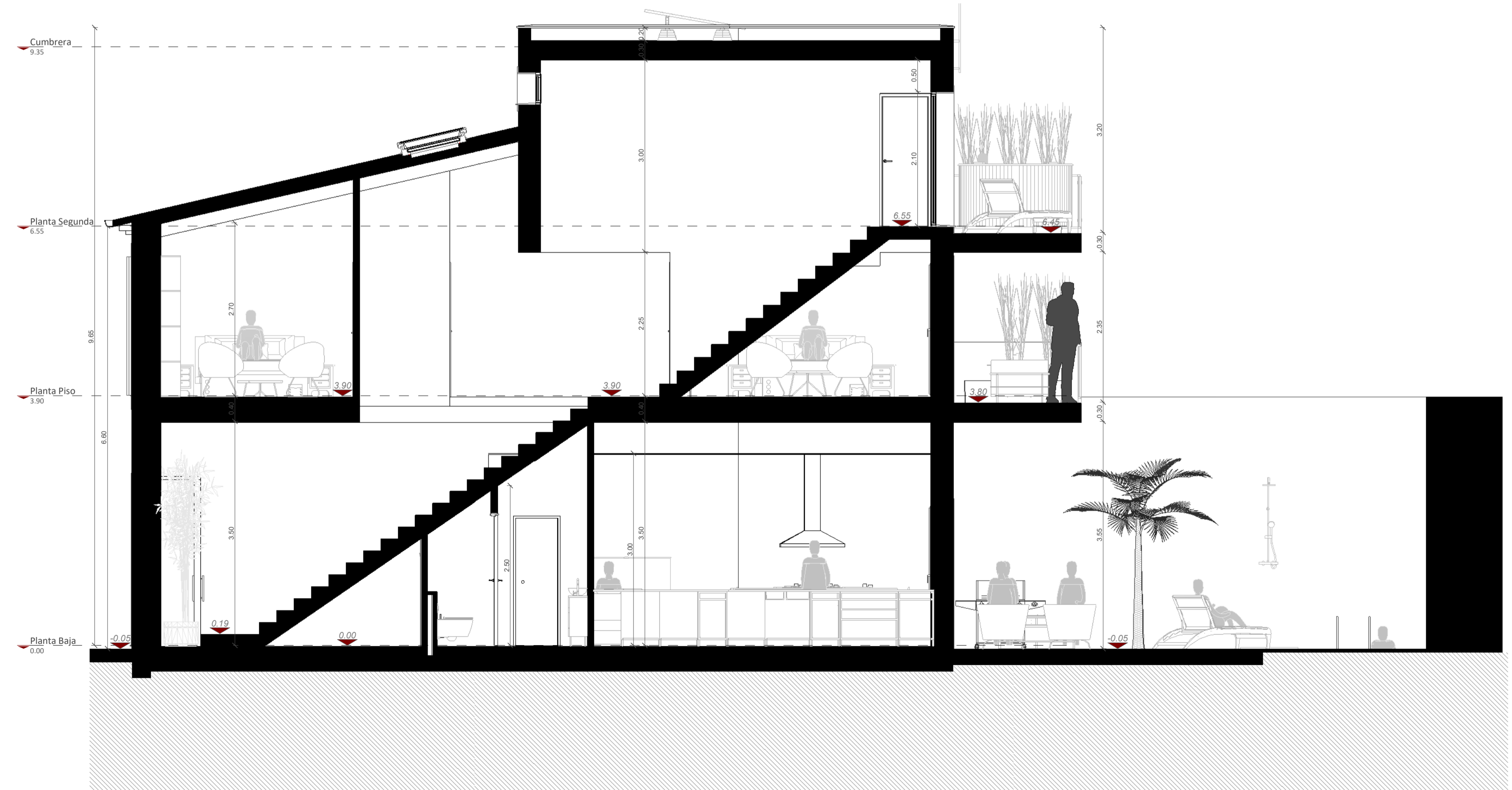
Sección C-C' 1:50
