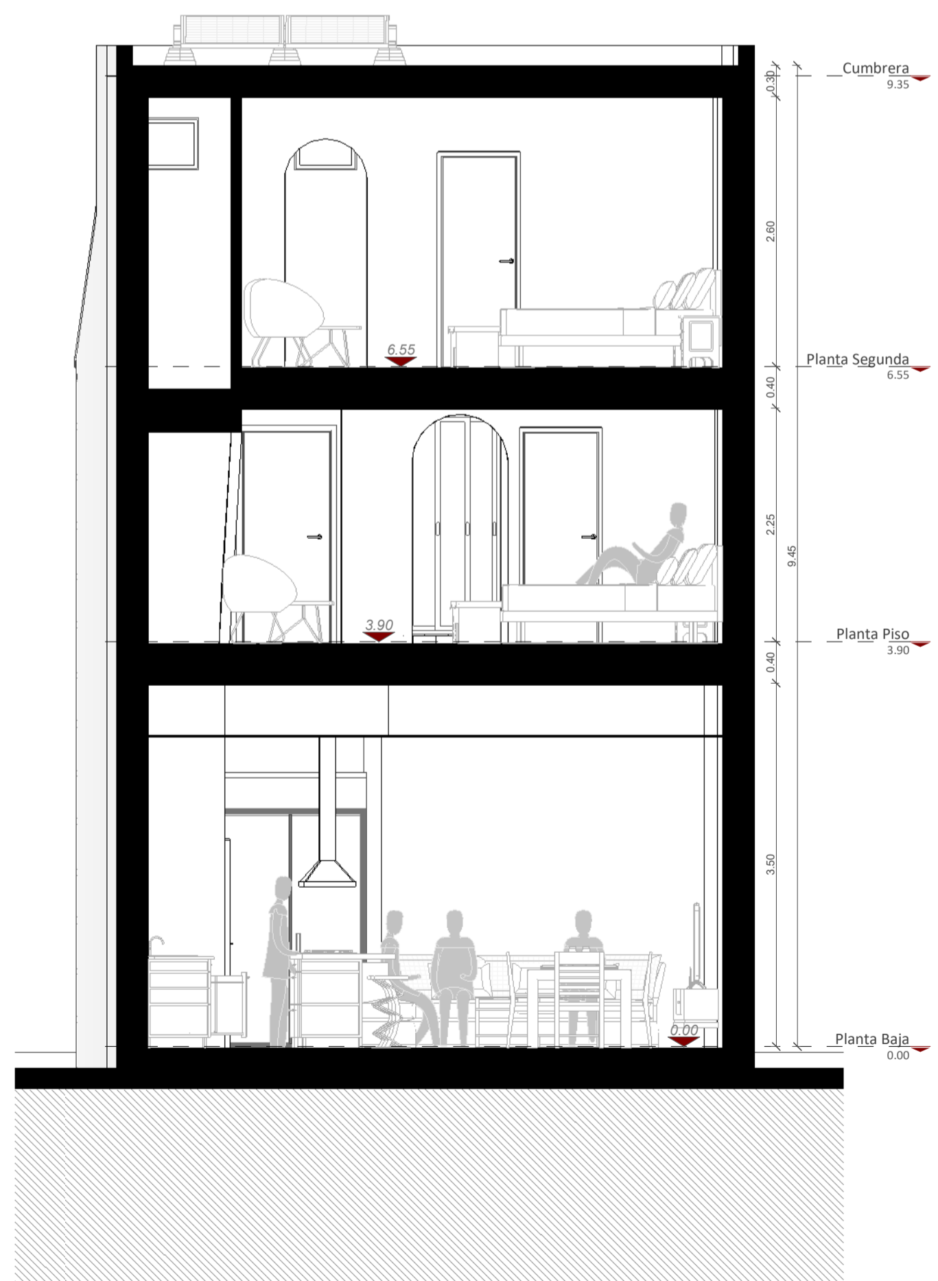
Sección A-A' 1:50
