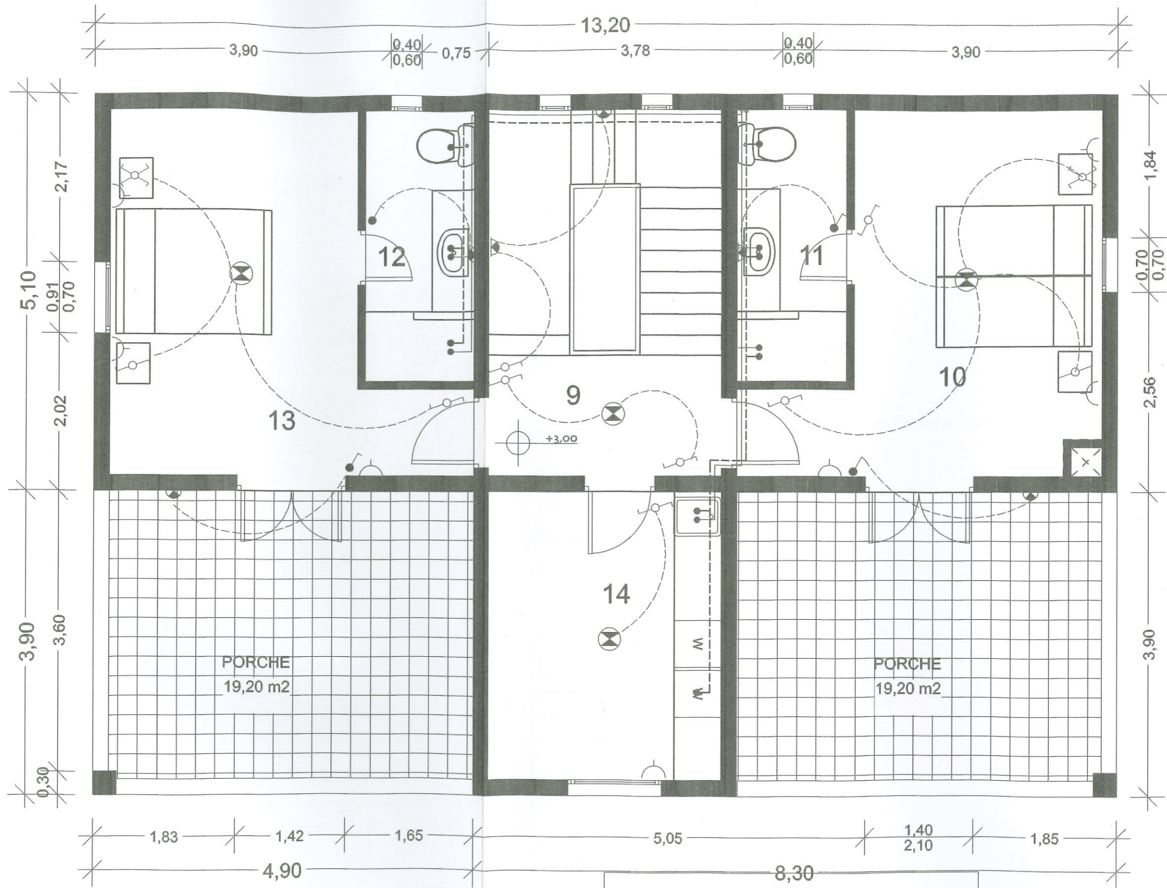
PLANTA PISO Esc. 1/50
