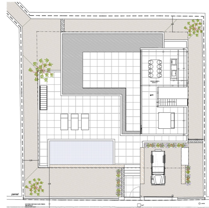
Dachgeschoss
